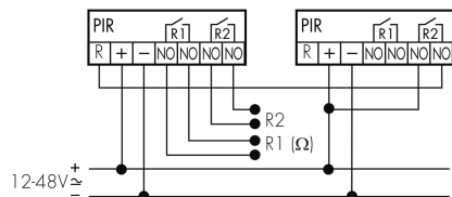
Funzionamento Master-Slave (Master in funzionamento Slave)
