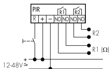
Funzionamento normale con tasto esterno
