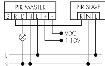
Fonctionnement Master-Slave
