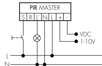
Fonctionnement normal avec bouton externe
