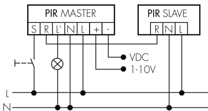
Fonctionnement Master-Slave avec bouton externe
