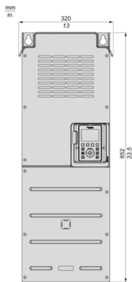
Variateurs sans capot supérieur IP21 Vues droite et avant
