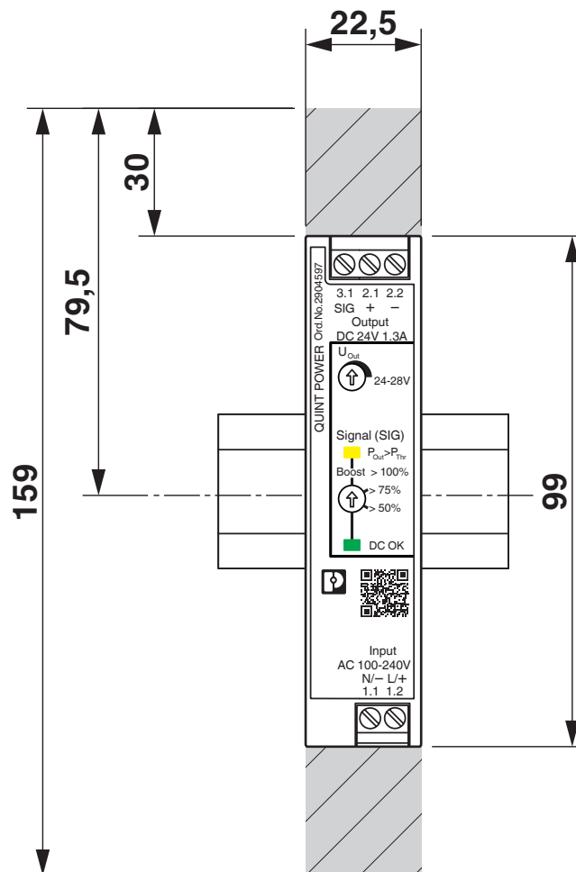
Disegno quotato
